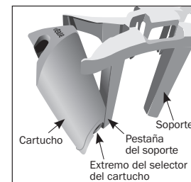
Detalle de la pestaña del soporte del cartucho
